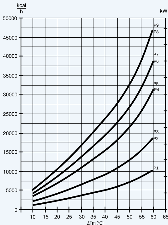
DIAGRAMMA DI RENDIMENTO PERFORMANCE DIAGRAM LEISTUNGSSCHAUBILD DIAGRAMME DE RENDEMENT
