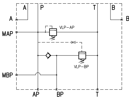
SCHEMA IDRAULICO TIPO 0
